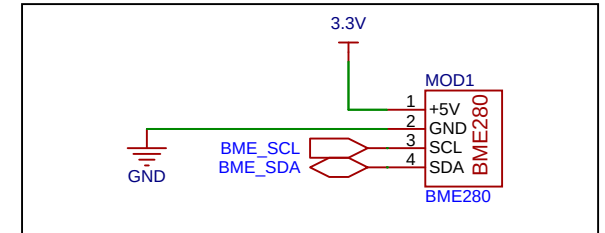
SENSOR DE PRESION, TEMPERATURA Y HUMEDAD BME280
