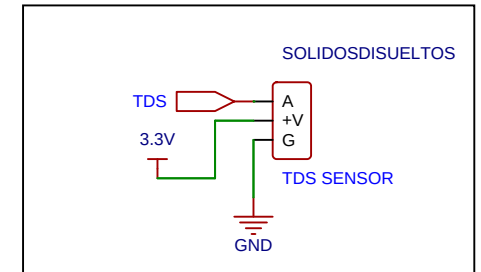
SENSOR DE SOLIDOS DISUELTOS TDS
