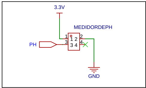
MEDIDOR DE PH
